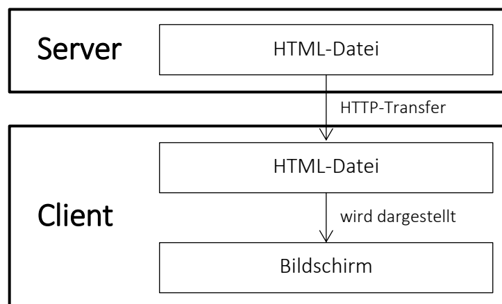
Abbildung 10: Statische Webseiten
