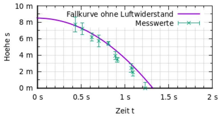
Abbildung 10: Graph des Falls ohne Luftwiderstand und Messpunkte beim Holzblock
