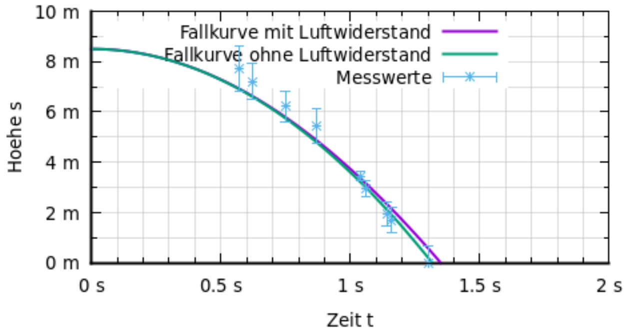
Abbildung 7: Graphen des Falls mit und ohne Luftwiderstand für den Tennisball
