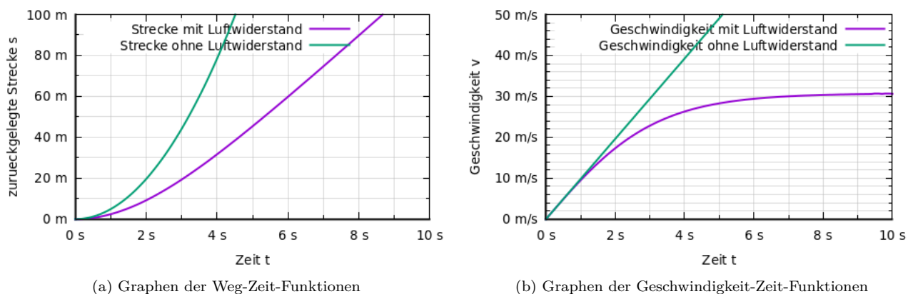
Abbildung 4: Graphische Unterschiede beim Fall mit und ohne Luftwiderstand
