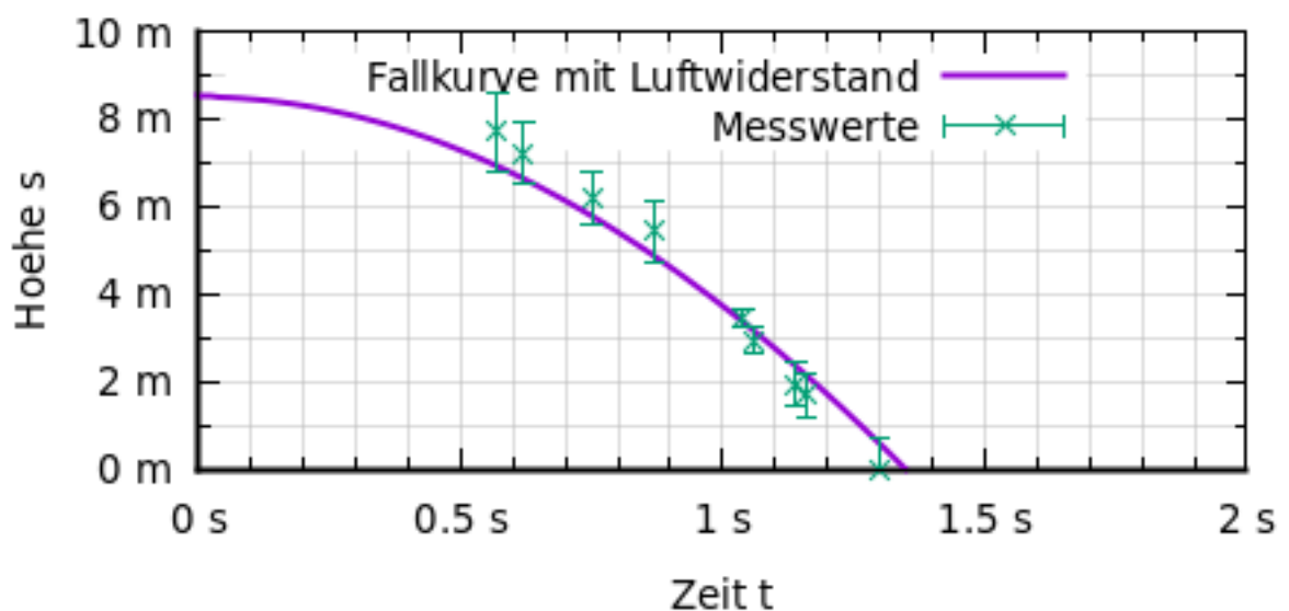
Abbildung 6: Graph des Falls mit Luftwiderstand für den Tennisball
