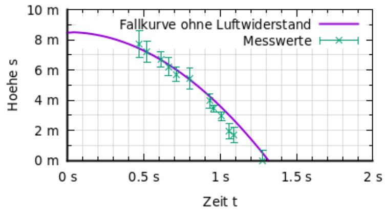
Abbildung 9: Graph des Falls ohne Luftwiderstand und Messpunkte beim Holzpfahl
